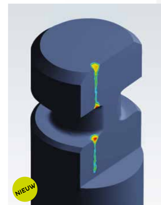
S201 L Pro en S201 XL Pro: De verdeling van het koppel over een groter oppervlak leidt tot minder vervorming van de gereedschapsrand en bovendien wordt de belasting van de asrand in de richting van het midden van de as verschoven. Op deze manier wordt vervorming van de as voorkomen.
